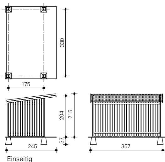
Typ 3100 mit beschichteten Stahl-Trapezprofilen.
